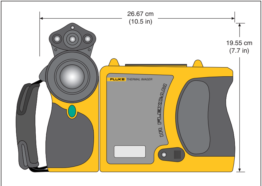
图 D-2. 热像仪尺寸 - 高度和宽度
